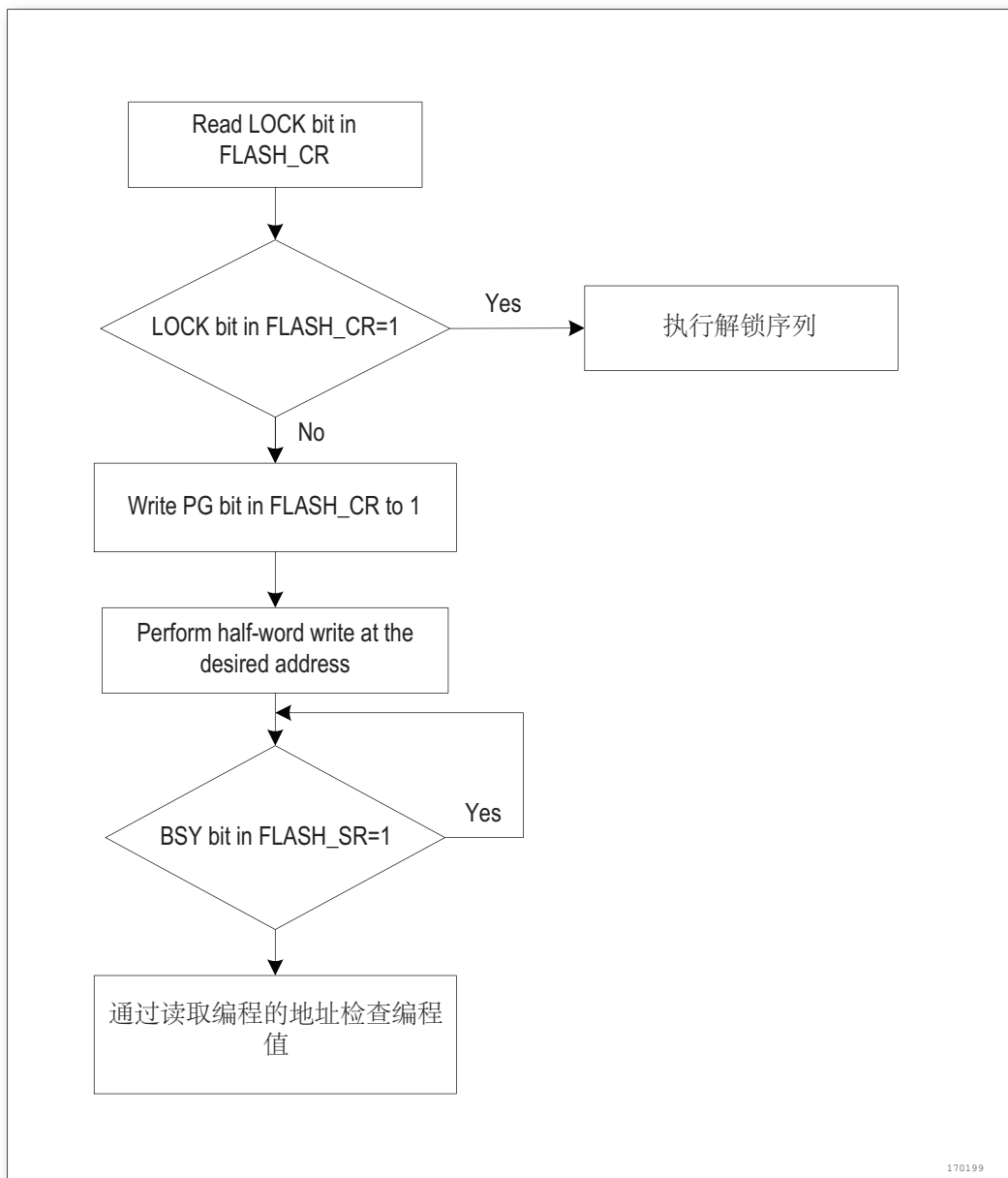
图 2. 编程流程
