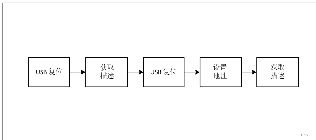
图 216. 枚举过程
