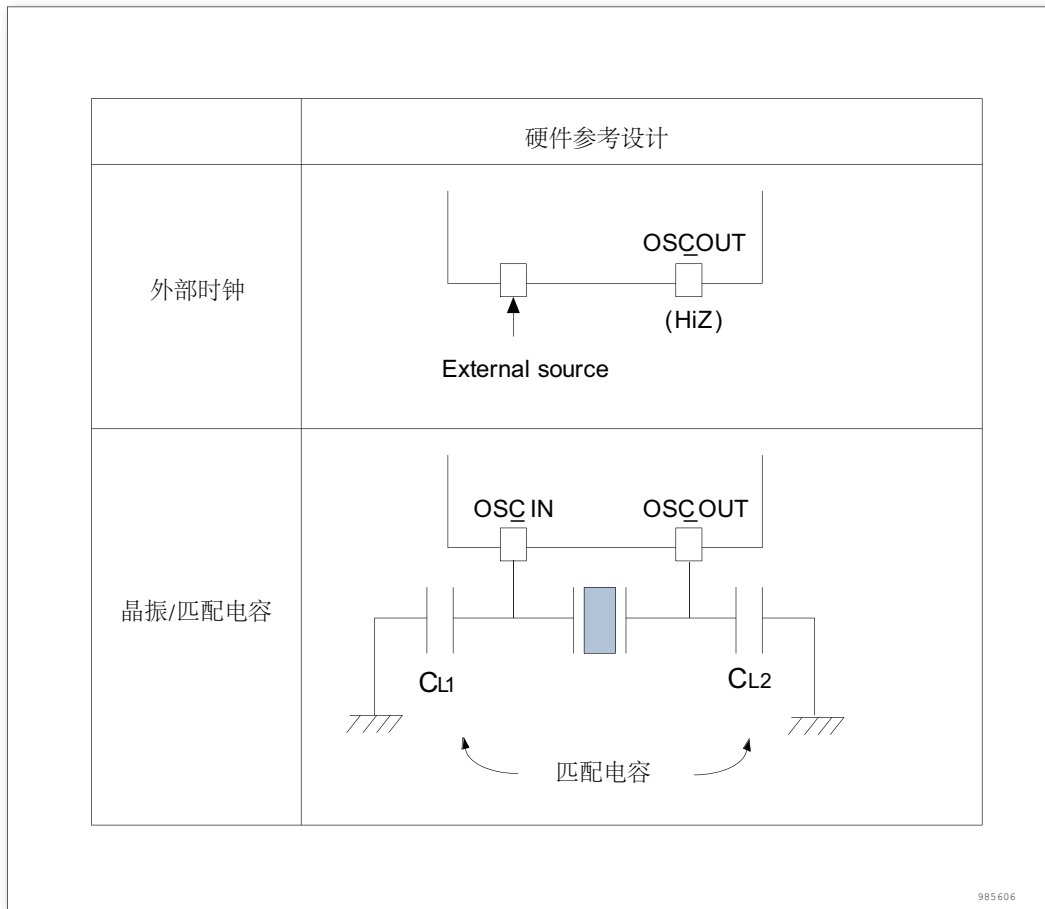
图 12. 时钟源
