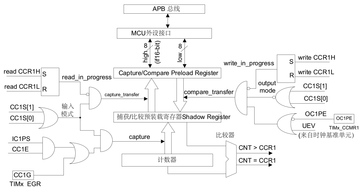
图 51. 捕获/比较通道 1 的主电路
