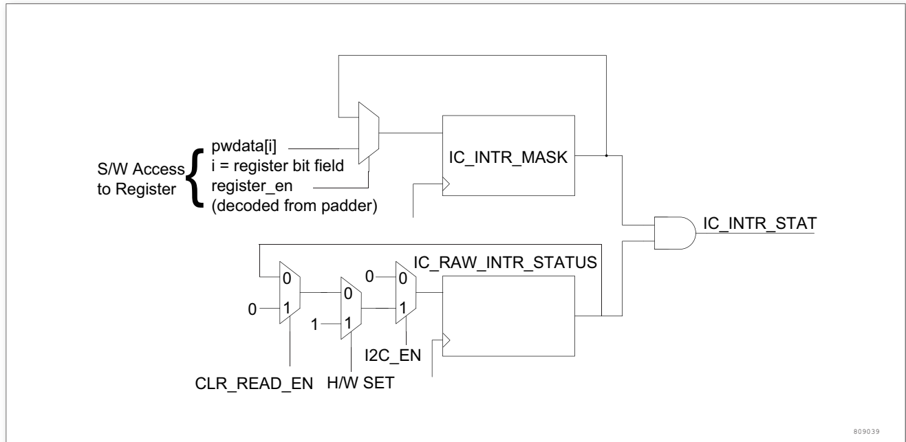
图 204. 中断机制
