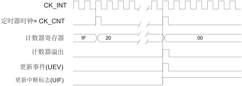
图 124. 计数器时序图，内部时钟分频因子为 N
