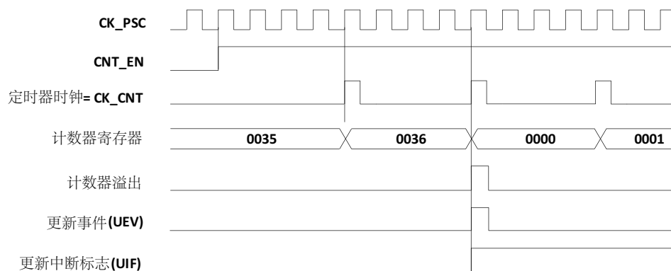
图 179. 计数器时序图，内部时钟分频因子为 4
