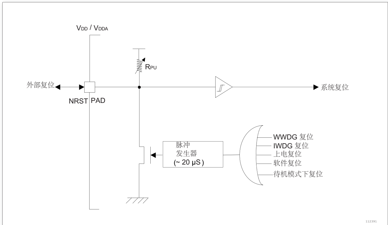
图 10. 复位电路
