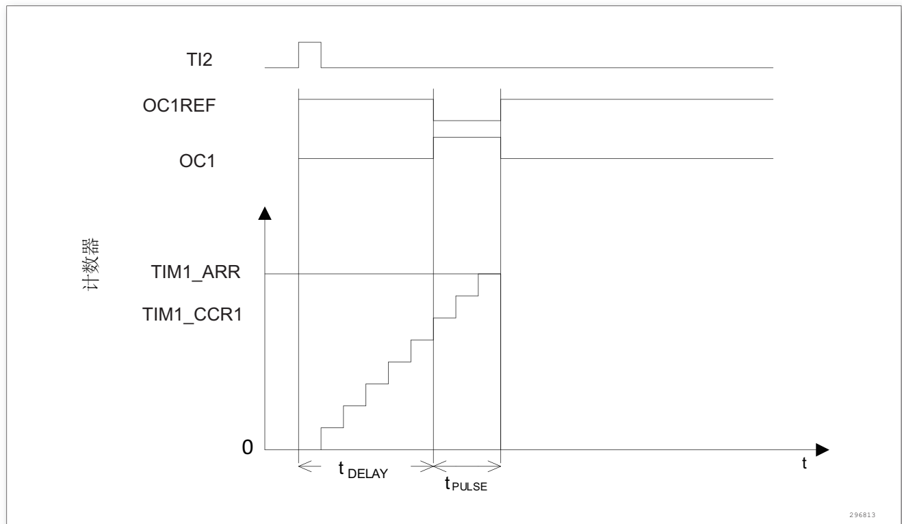
图 110. 单脉冲模式的例子
