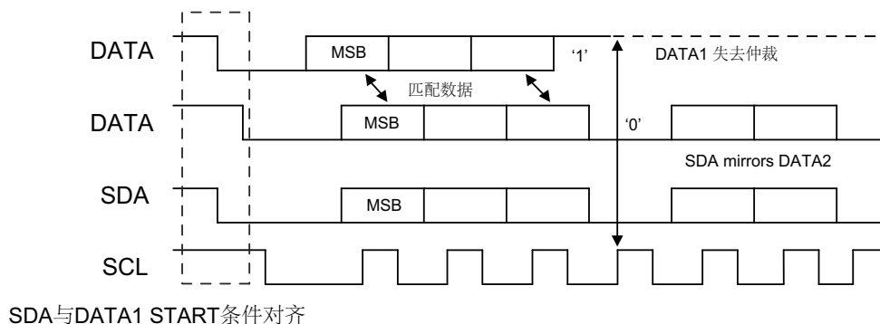
图 221. 多个主机仲裁
