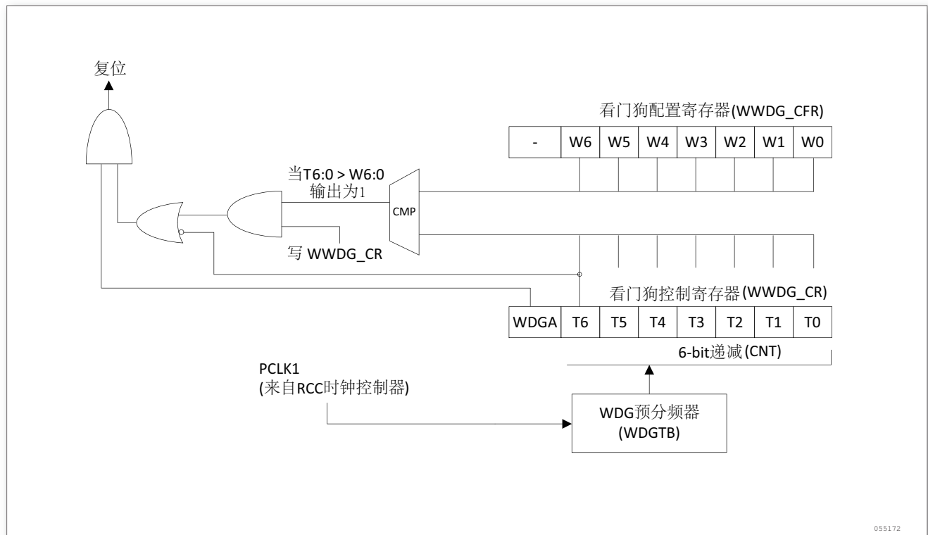
图 207. 看门狗框图
