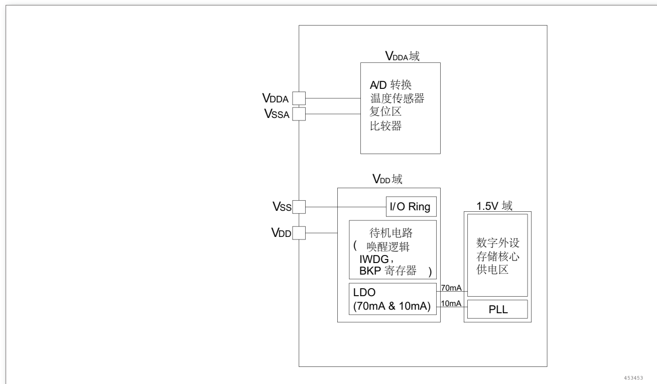
图 7. 电源框图
