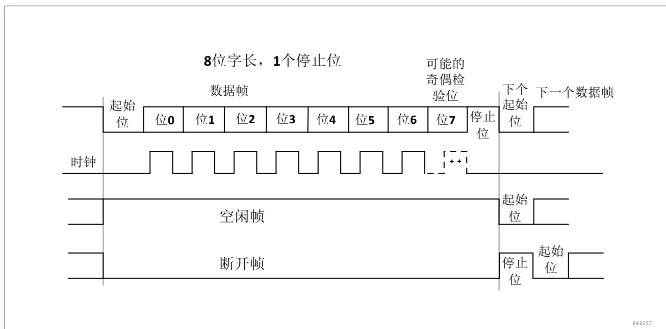
图 227. UART 时序
