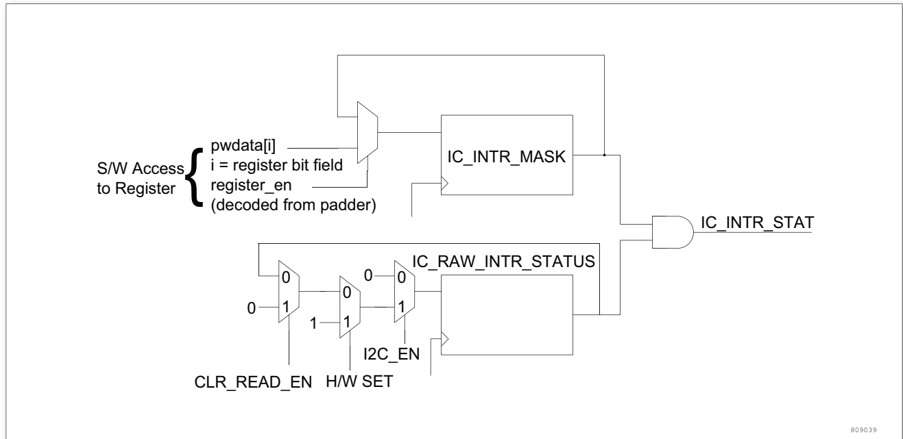
图 225. 中断机制
