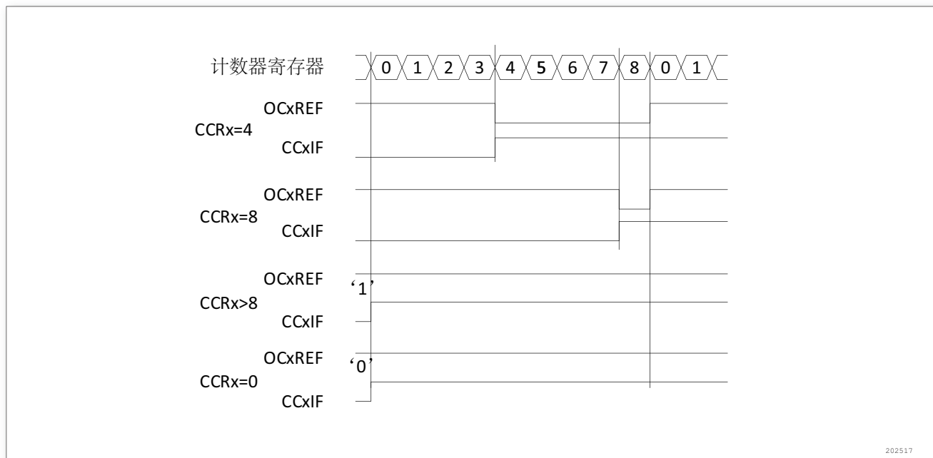
图 200. 边沿对齐的 PWM 波形 (ARR = 8)
