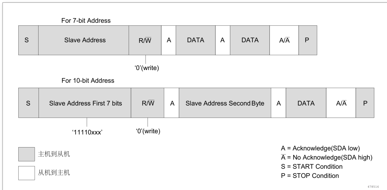
图 215. 主发送协议
