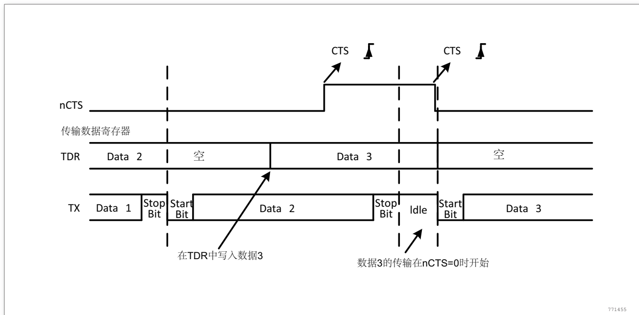
图 232. CTS 流控制
