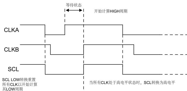
图 222. 多个主机时钟同步
