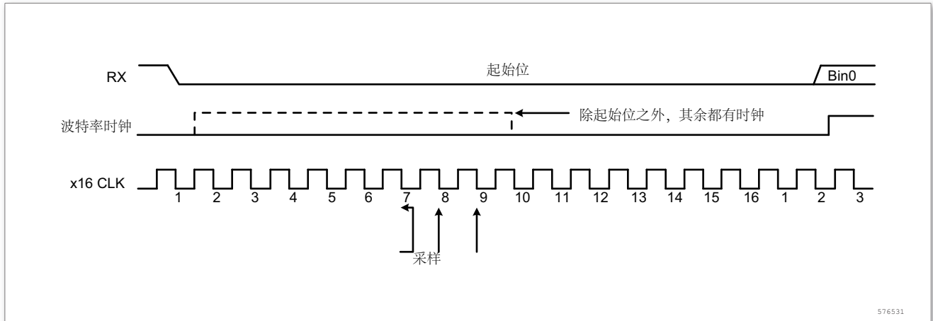
图 229. RX 引脚采样方案
