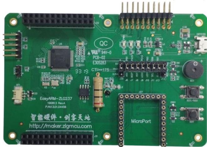
图 1.1 EasyARM-ZLG237 开发平台
