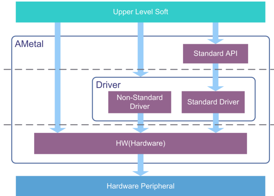
图 2.1 AMetal 框架
