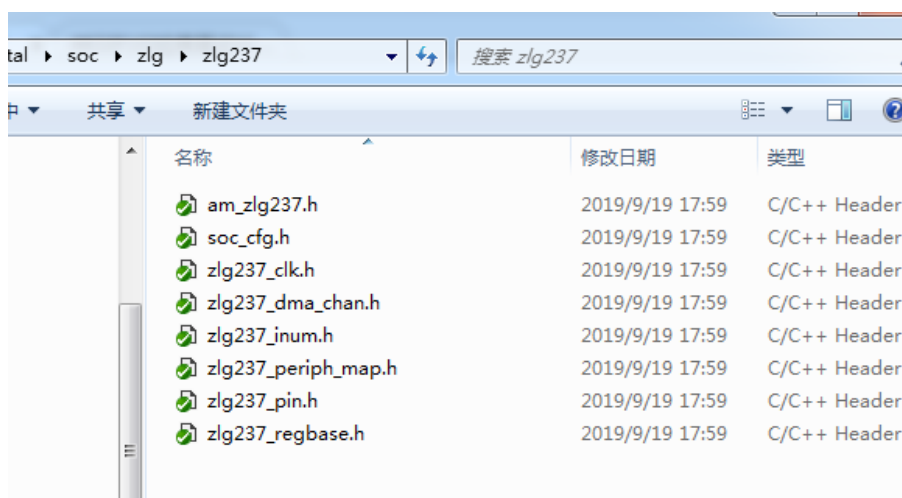
图 2.8 soc 目录
