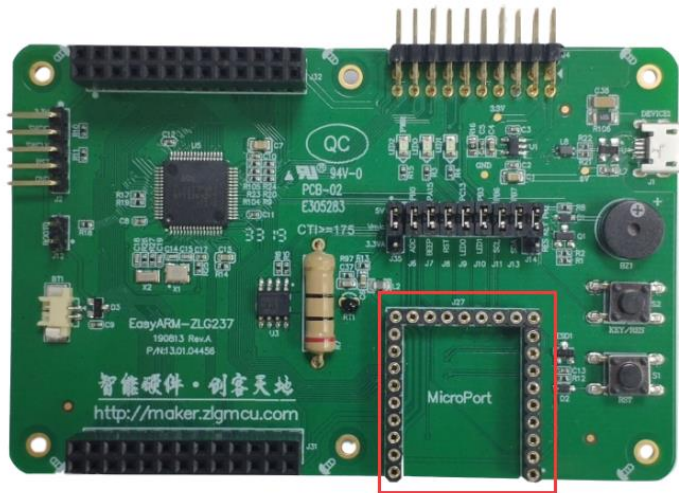
图 6.1 EasyARM-ZLG237 MicroPort
