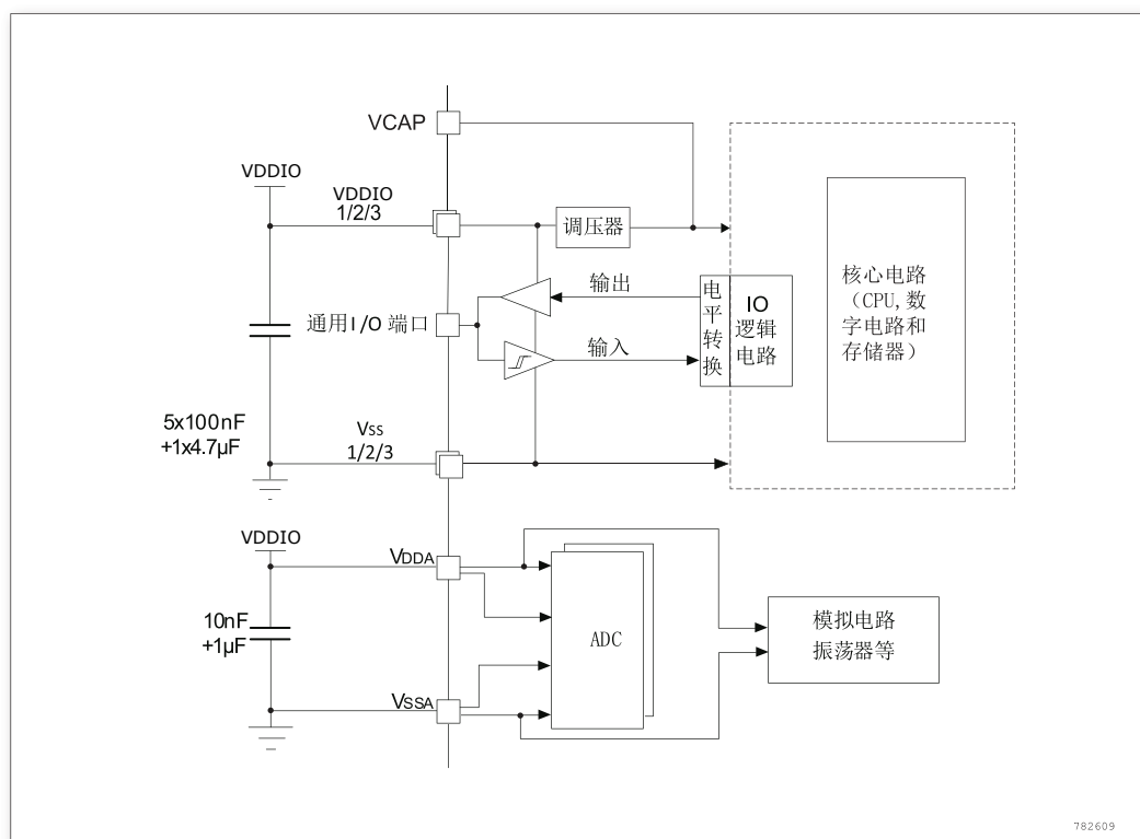
图 7. 供电方案
