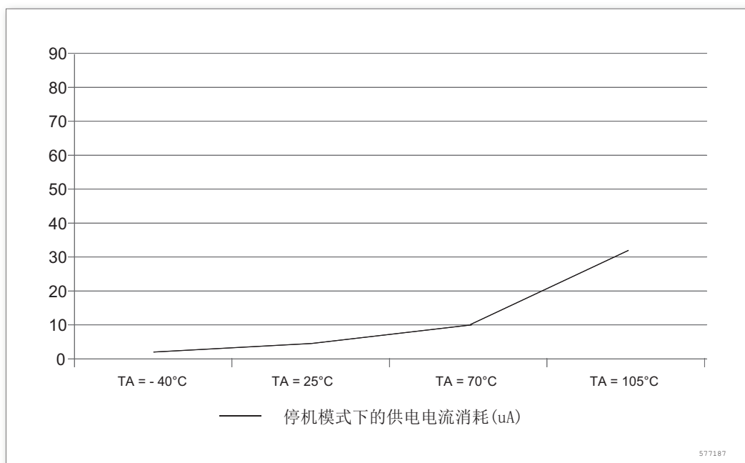
图 4. 待机模式下的典型电流消耗在 V_{DD} = 3.3\text{V} 时与温度的对比
