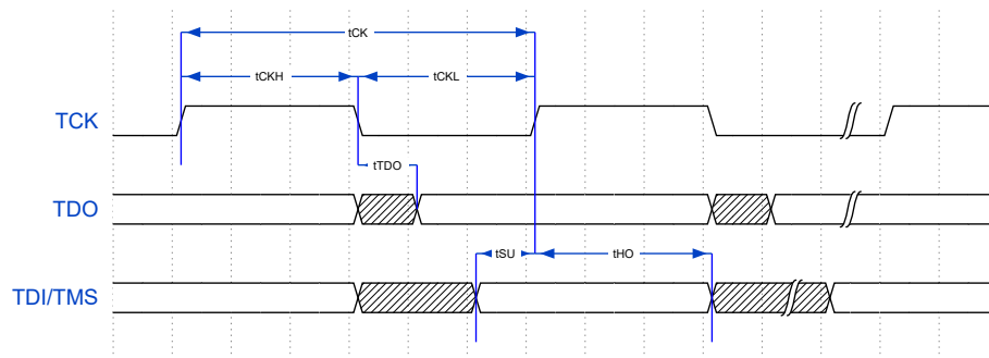
图 7: JTAG 时序图
