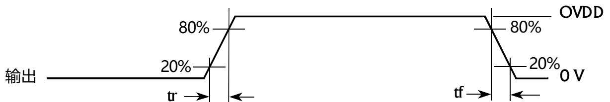
图 9: I/O AC 特性
