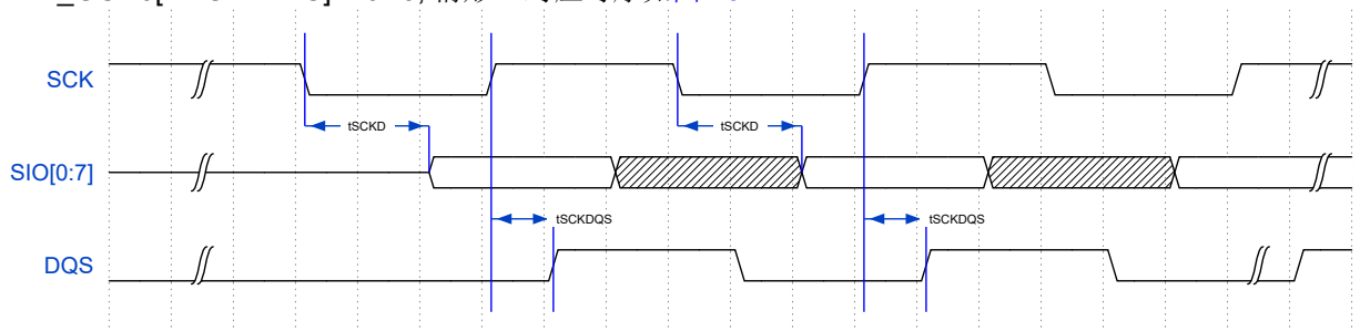
图 13: XPI SDR 模式的输入时序 (XPI_GCR0[RXCLKSRC] = 0X3, 情形 2)
