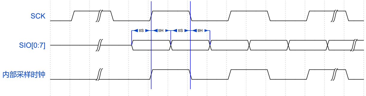
图 12: XPI DDR 模式的输入时序 (XPI_GCR0[RXCLKSRC] = 0X0,0X1)
