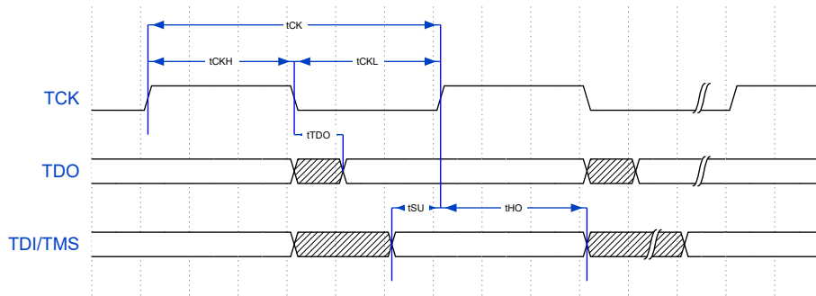
图 8: JTAG 时序图
